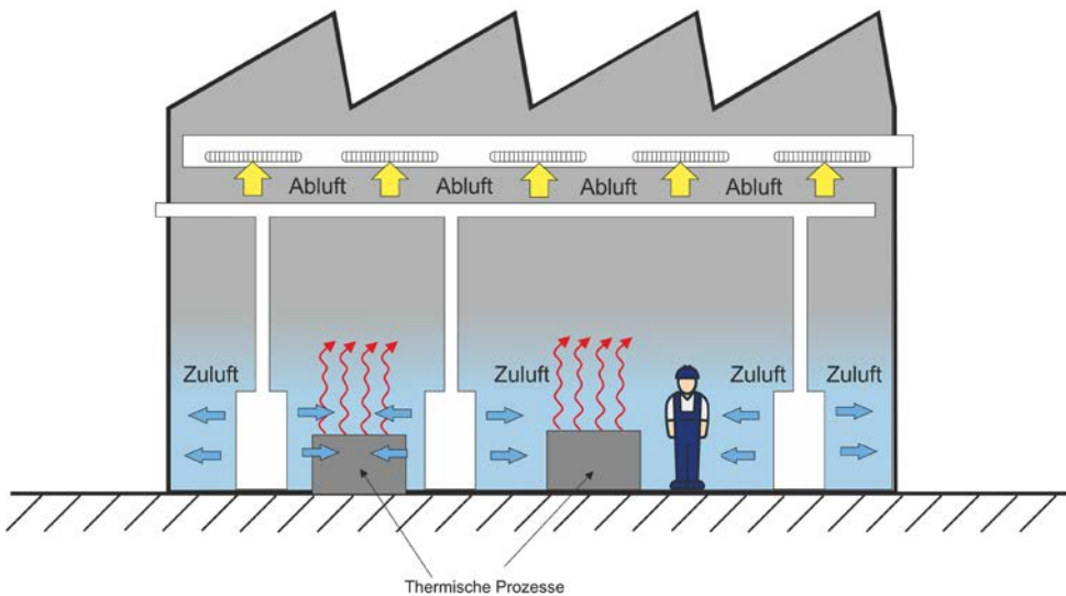
Abb. 10 Prinzip Schichtlüftung
